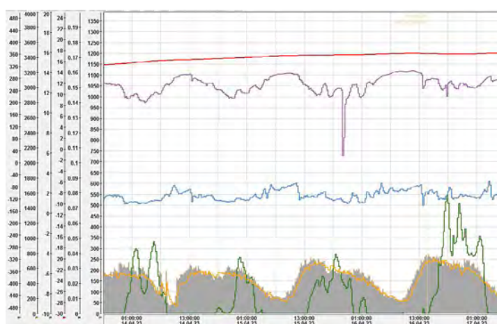
Abbildung 5: Trendkurven der Nitrifikation Abwassertemperatur [°C] (rot) RedOx-Potenzial [mV] (violett) Ammoniumfracht Zulauf Schwachlast [kg/h] (gelb) O 2 -Konzentration [mg/l] (blau) N 2 O-Konzentration [mg/l] (grün) Abwassermenge Ablauf GWK [m 3 /s] (grau) Quelle: StEB Köln
