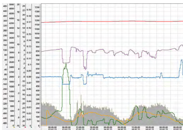
Abbildung 4: Trendkurven der Variokaskade Abwassertemperatur [°C] (rot) RedOx-Potenzial [mV] (violett) O 2 -Konzentration [mg/l] (blau) Ammoniumfracht Zulauf Schwachlast [kg/h] (gelb) N 2 O-Konzentration [mg/l] (grün) Abwassermenge Ablauf GWK [m 3 /s] (grau) Quelle: StEB Köln
