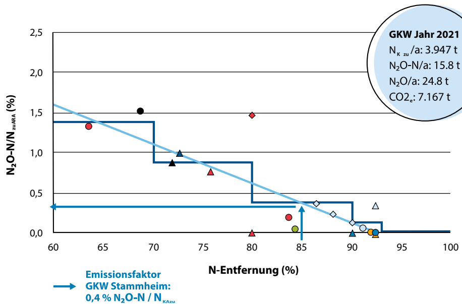
Abbildung 2: Emissionsfaktor N 2 O-N/N KAZU -KA in Abhängigkeit der N-Entfernung Quelle: nach Studie "ReLaKo" der TU Wien 2015 Die Studie untersuchte verschiedene Kläranlagen. Die unterschiedlichen Formen im Diagramm stellen die Ergebnisse der Kläranlagen dar.
