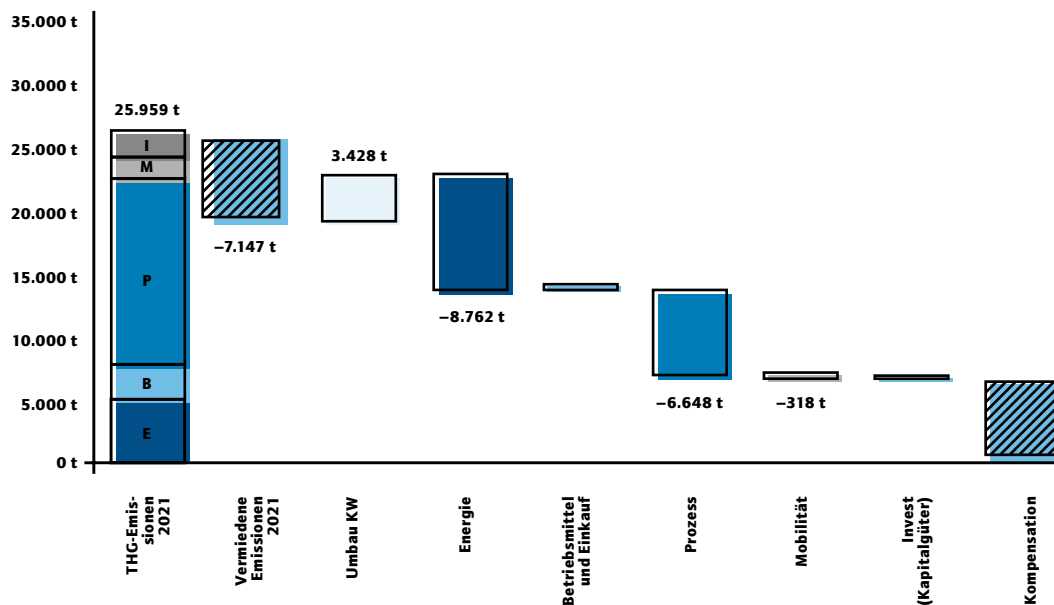
Abbildung 4: CO 2 -Roadmap-Maßnahmen mit den Zielbeiträgen je Handlungsfeld Quelle: StEB Köln
