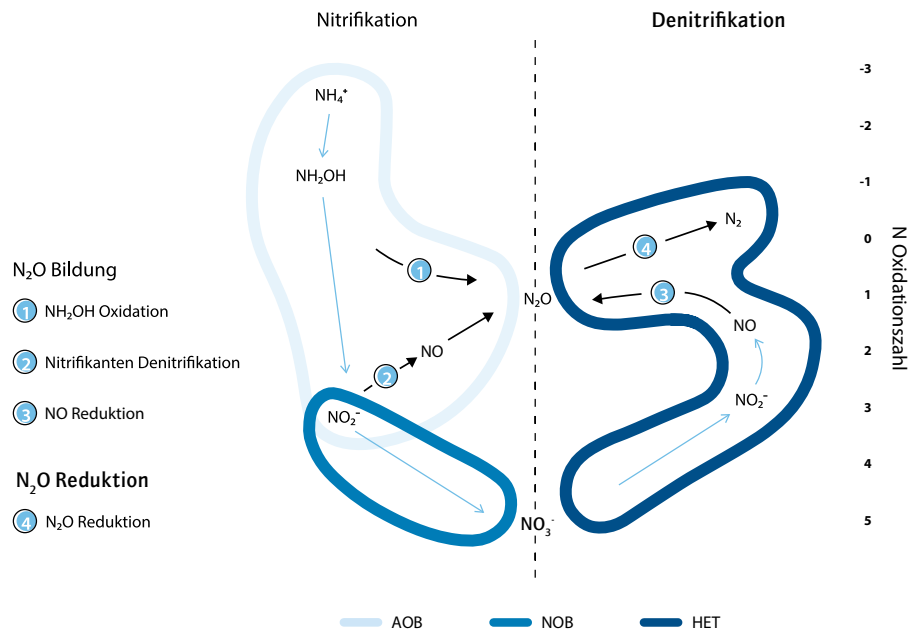
Abbildung 1: N 2 O-Bildungswege und Reduktionswege innerhalb der Nitri- und der Denitrifikation Quelle: Gruber, Wenzel et al 2022
