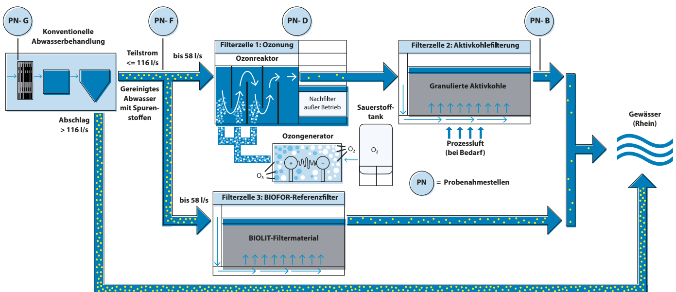
Abbildung 1: Fließbild der Pilotanlage im Projekt RedOxA / Quelle: StEB Köln Bild linke Seite: Klärwerk-Rodenkirchen / © StEB Köln, Sabine Grothues
