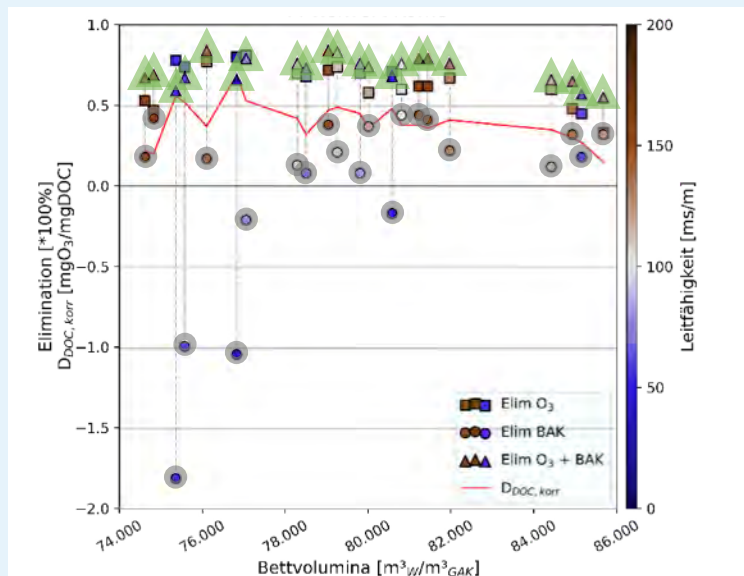
Abbildung 4: Wirkungsgrad für Aktivkohle bei höherer Standzeit Quelle: StEB Köln
