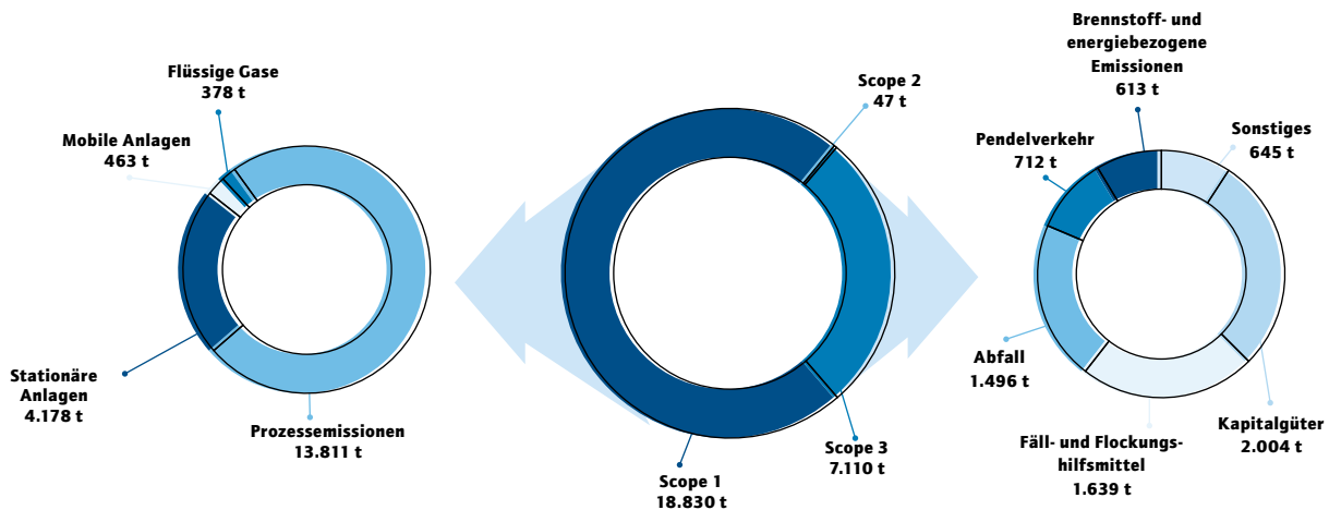
Abbildung 3: CO 2 e-Emissionen mit Fokusbetrachtung Scope 1 und Scope 3 Quelle: StEB Köln, Roadmap zur Erreichung der Klimaneutralität der StEB Köln bis 2030
