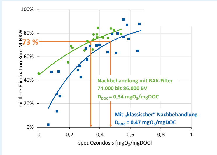
Abbildung 3: Ozonbedarf mit Nachbehandlung Blähton (Projekt AdOx) bzw. Aktivkohle (RedOxA) Elimination gemittelt für die Stoffliste laut Kompetenzzentrum Mikroschadstoffe NRW (KomM NRW) Quelle: StEB Köln
